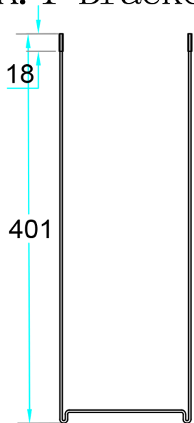
A. 1 Bracket L401*135
