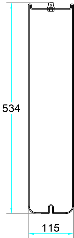
A. Bracket L534*115
